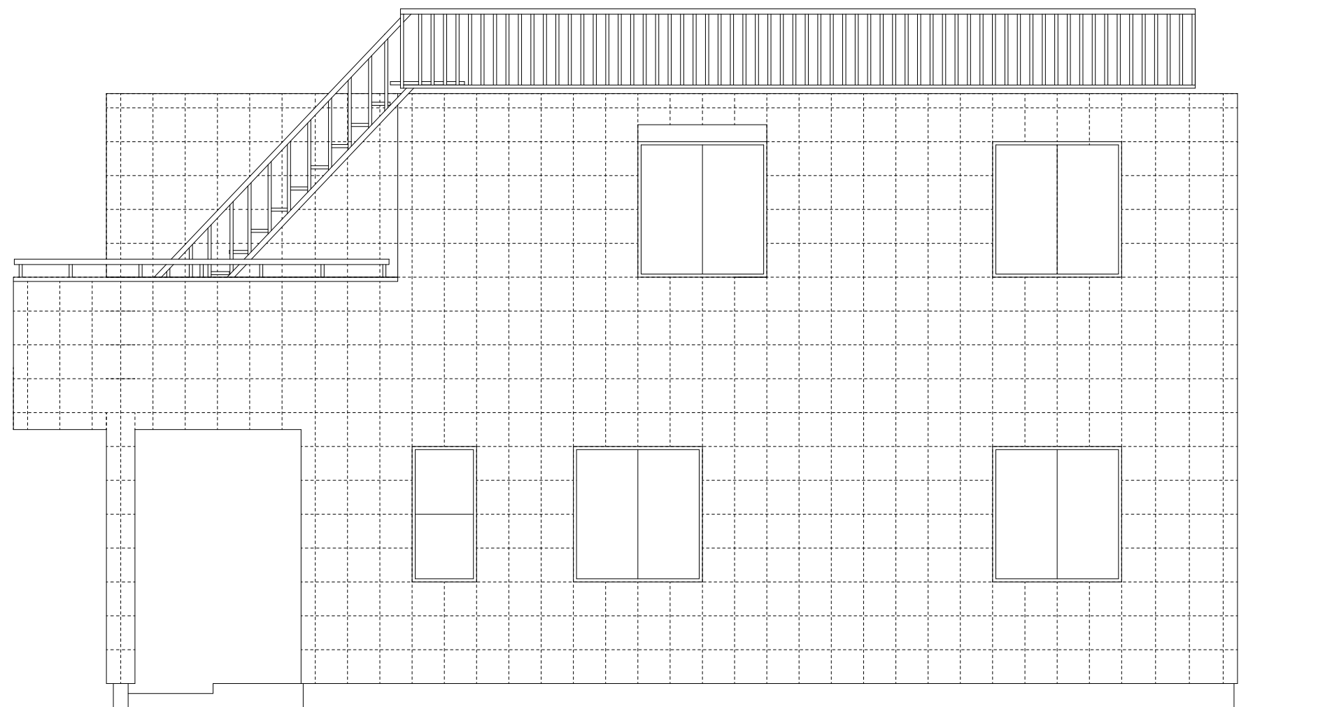
南側立面図
